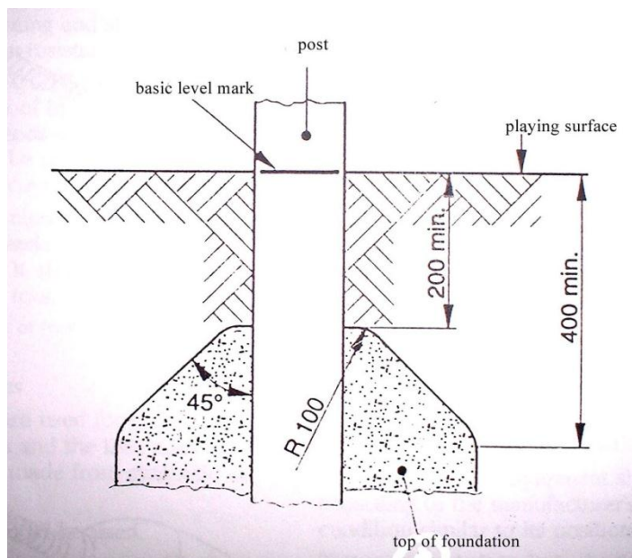
รูปที่ 16 ตัวอย่าง การจัดทำฐานรากเพื่อติดตั้งเครื่องเล่นอย่างมีเสถียรภาพ
